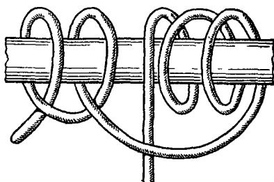
Рис. 59. Верблюжий узел
