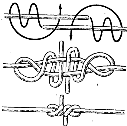
Рис. 34. Змеиный узел
