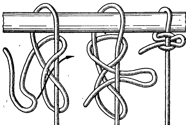
Рис. 102. Курбёрский узел
