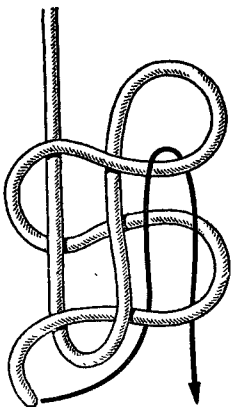
Рис. 137. Кордовый узел
