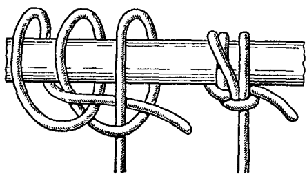
Рис. 58. Щучий узел
