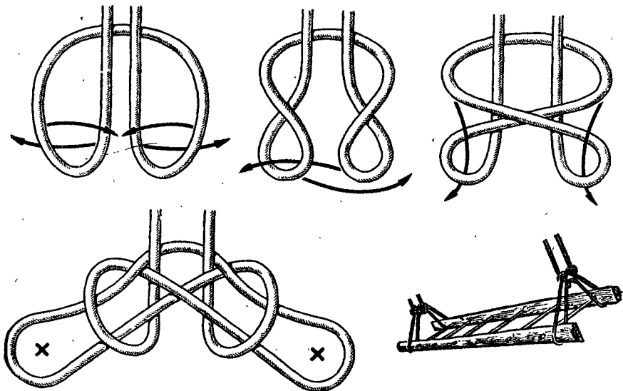
Рис. 78. Боцманский узел (испанский беседочный)
