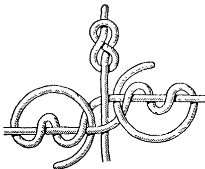
Рис. 132. Поводковый на основе змеяного узла
