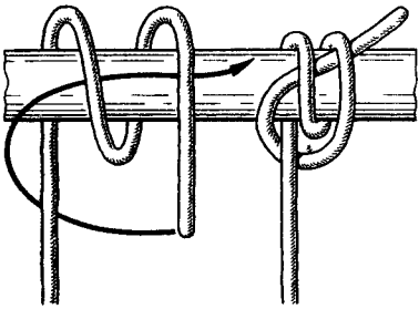
Рис. 55. Гафельный узел
