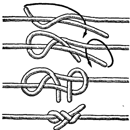
Рис. 32. Пакетный узел
