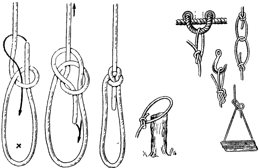
4 Рис 76 Беседочный узел
