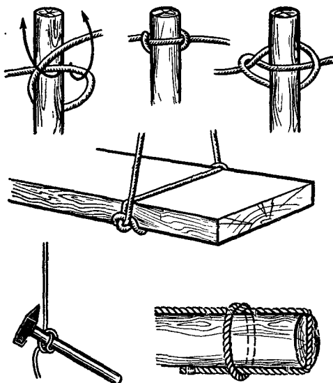
Рис. 110. Сваечный узел
