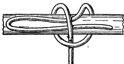
Рис. 99. Шлюпочный узел
