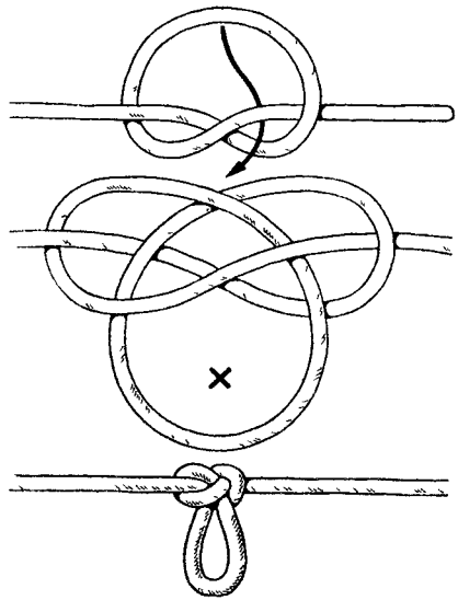
Рис 75 «Травяная» петля
