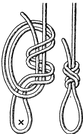
Рис. 67. Жилковая петля
