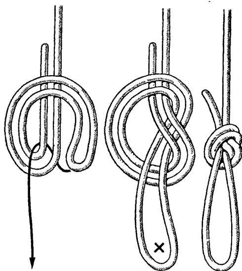
Рис. 66. Дубовая петля
