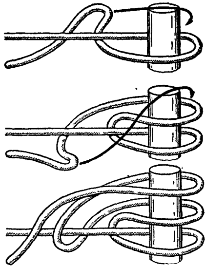
Рис. 18. Буксирный узел
