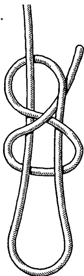
Рис. 83. Скользящая восьмерка
