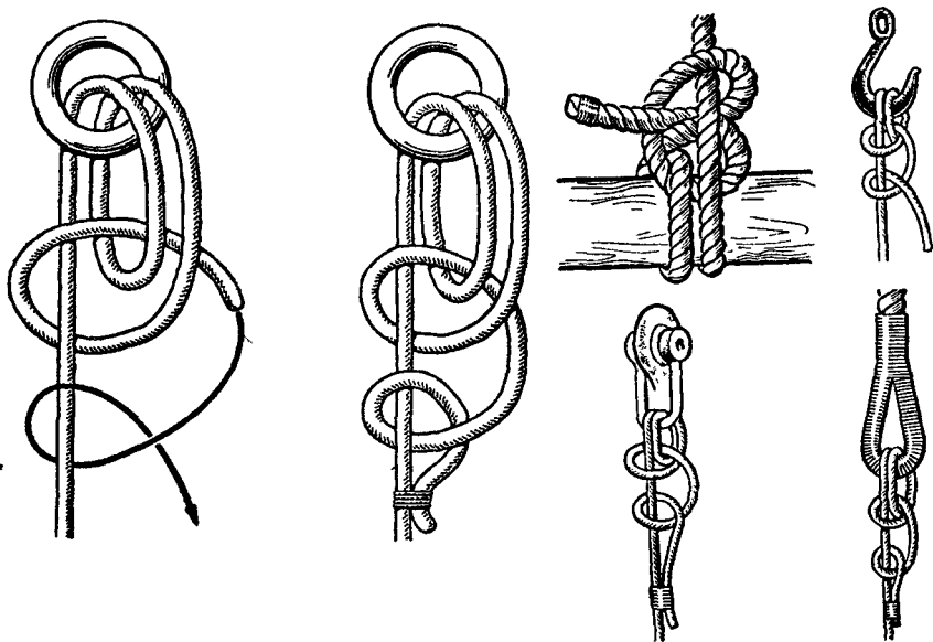
▲ Рис. 15. Рыбачий штык (якорный узел)
