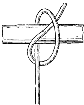
Рис. 44. Самозатягивающийся узел
