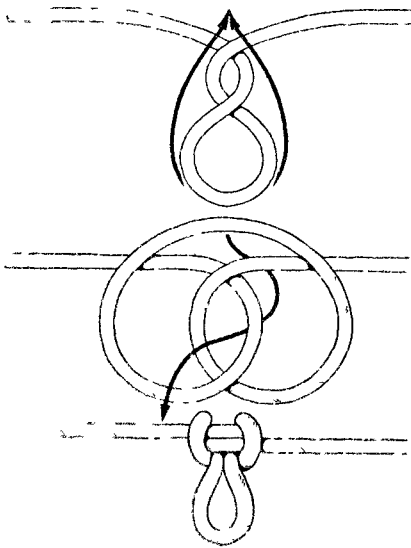
Рис 74 Фидовая петля
