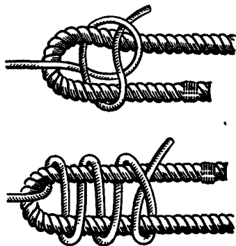
Рис. 40. Докерский узел (справа внизу — другой вариант узла)
