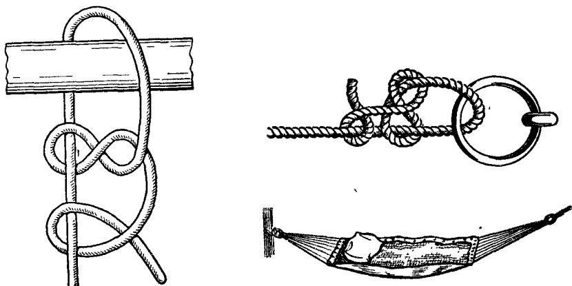
Рис. 11. Кочный штык
