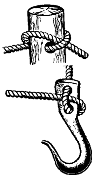
Рис. 44. Самозатягивающийся узел
