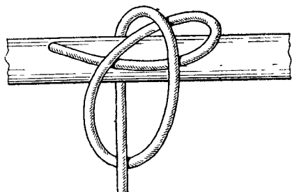
Рис 98 Развязывающийся самозатягивающийся узел
