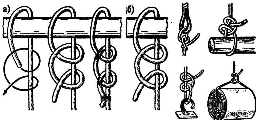
Рис 10 Простой штык
