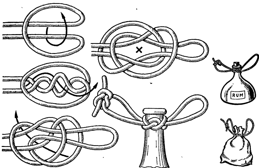
Рис. 111. Амфорный узел
