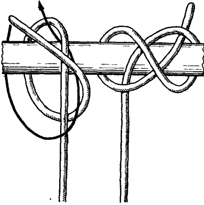
Δ Рис. 50. «Констриктор»
