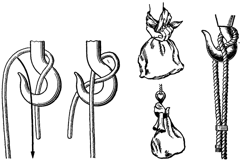
Рис. 105. Гачный узел
