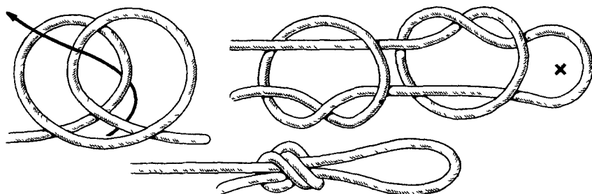
Рис 72 Рыбачья петля
