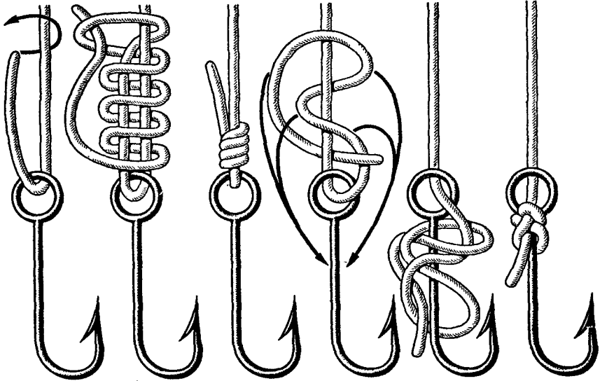
Рис. 127 Акулий узел
