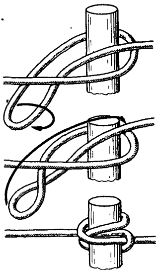
Рис. 64. Битенговый узел
