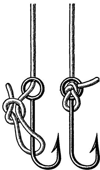
Рис. 123. Черепаший узел
