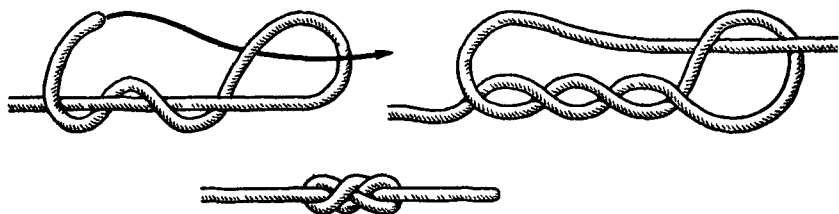
Рис. 4 Стивидорный узел
