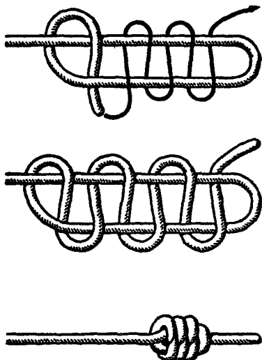
Рис. 7. Множественная восьмерка
