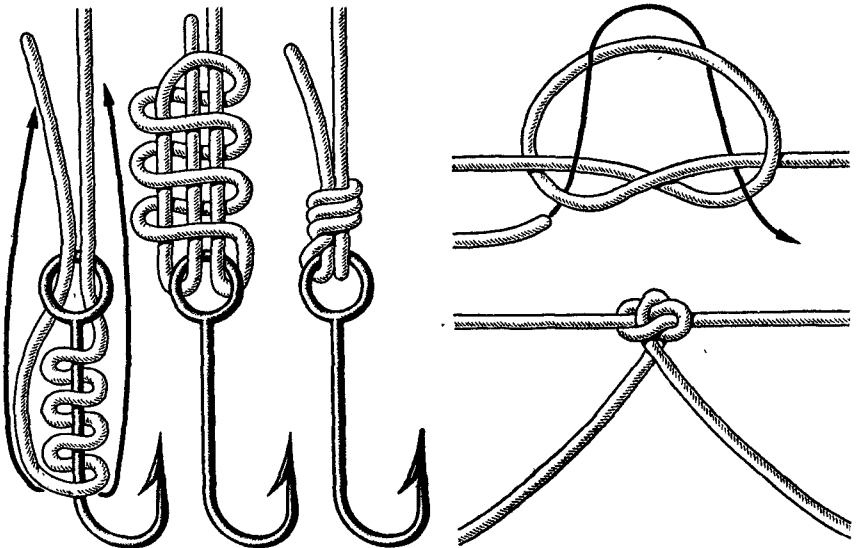
Рис 129. Тунцовый узел
