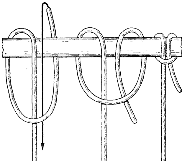
Рис. 46. Коровий узел
