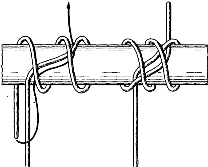
Рис. 51. Двойной «констриктор»
