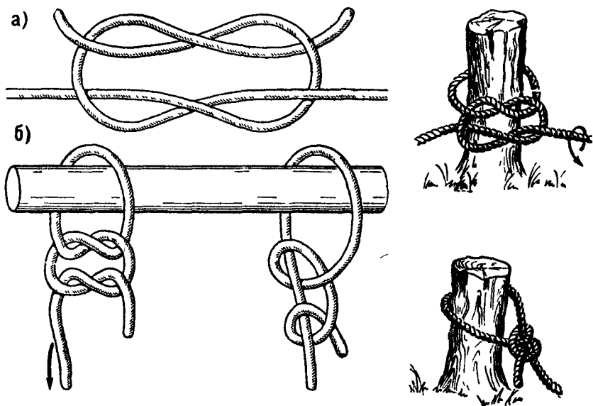
Рис 23 Бабий узел:
