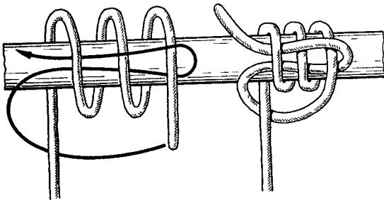
Рис. 57. Фаловый узел
