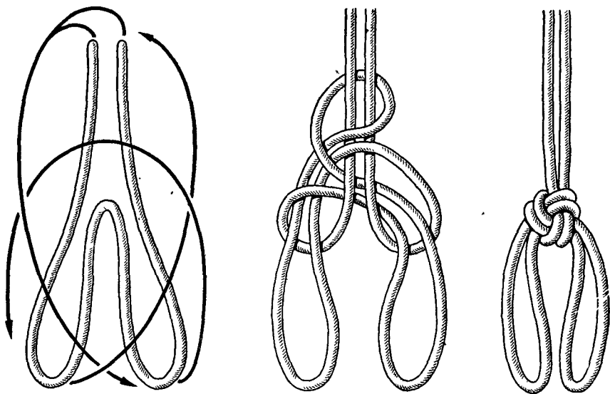
Рис. 139. Тройной плетеный узел
