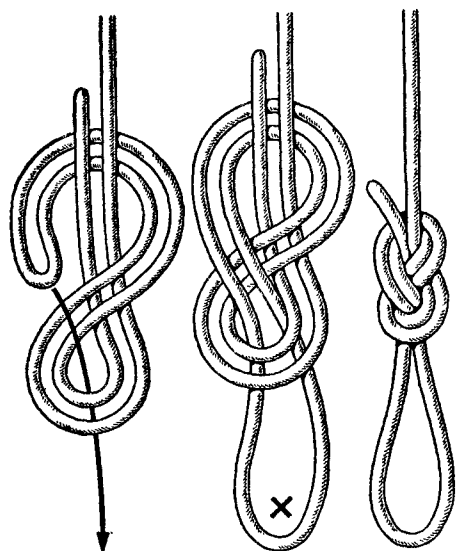
Δ Рис. 68 Фламандская петля
