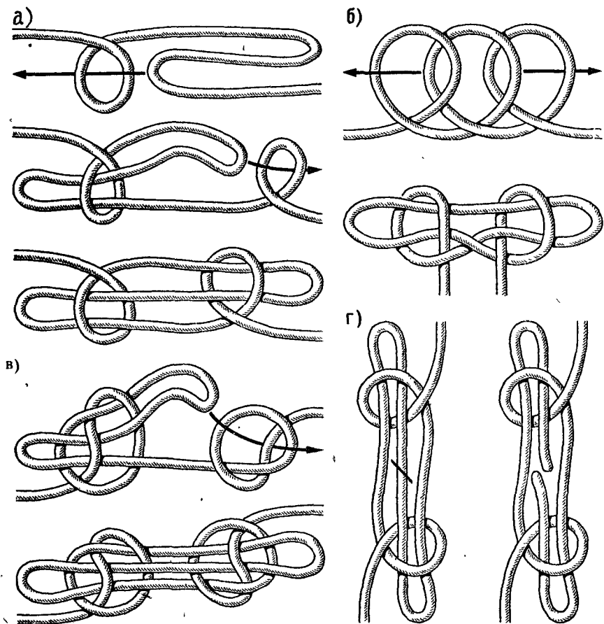
Рис. 113. «Баранья нога»:
