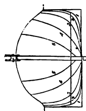
Fig. 3.—Body Plan.
